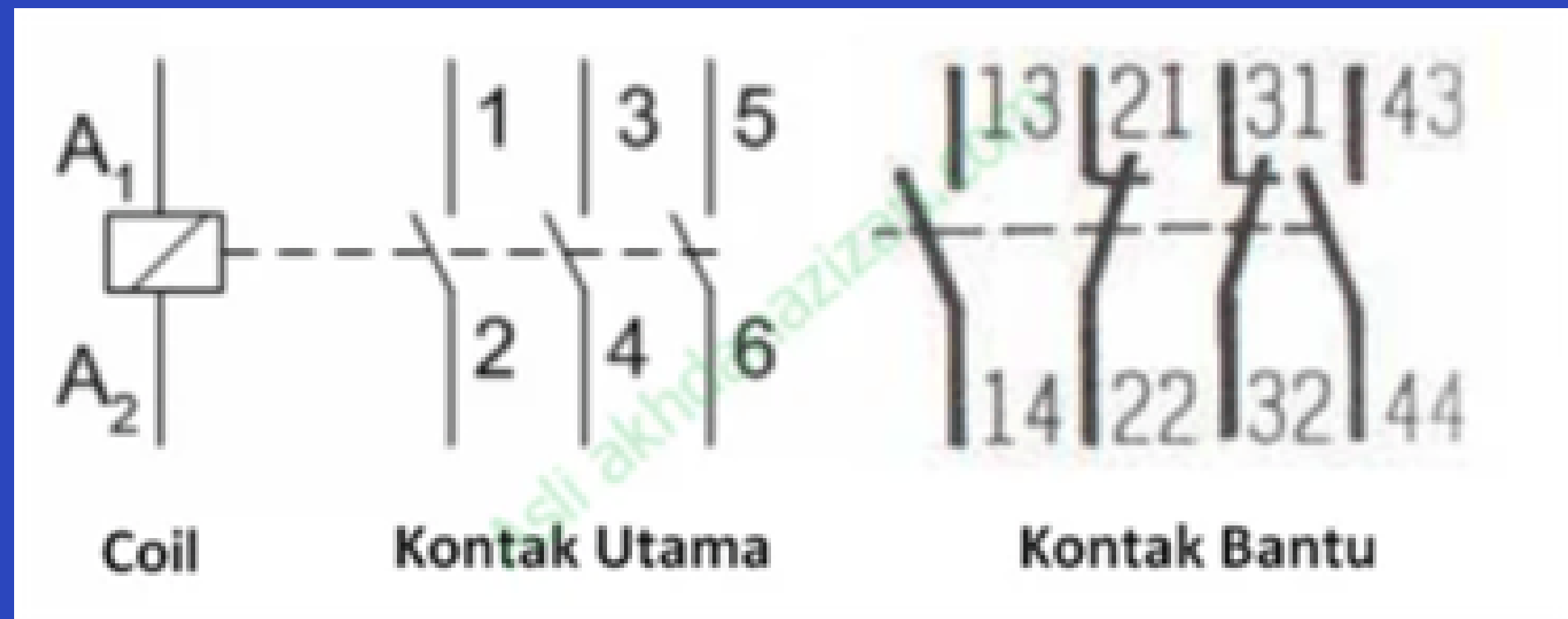
Simbol Kontaktor
